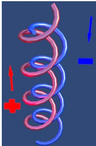
Рис.7.Предлагаемые формы электрона
