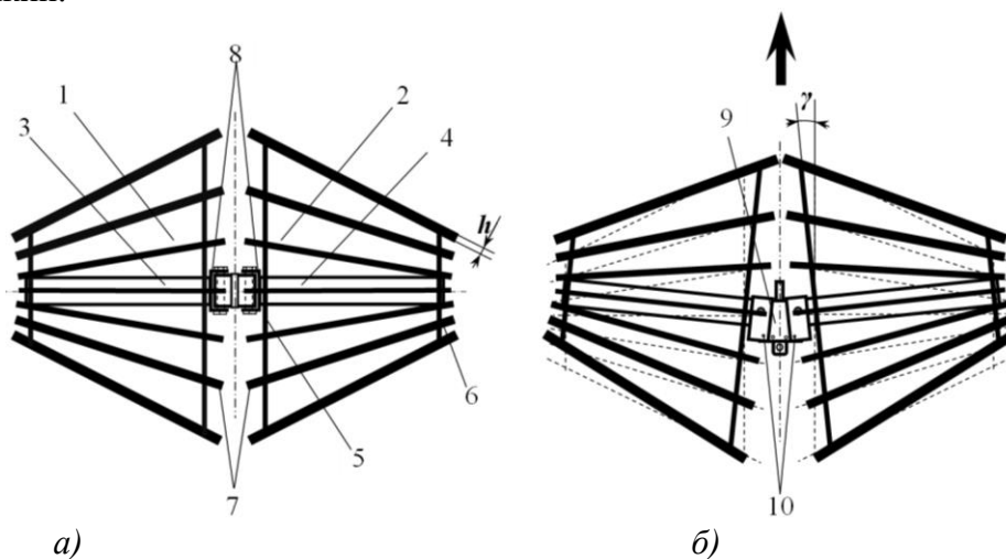
а) олтидан кўриниши; б) тепасидан кўриниши
